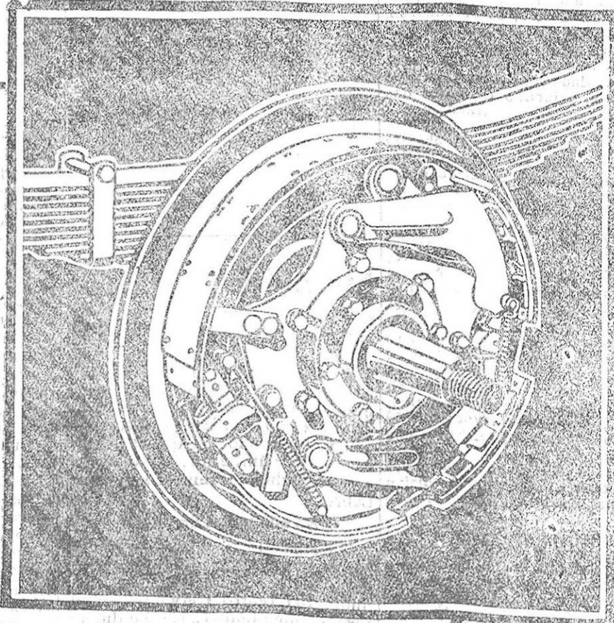
Sección de un freno delantero
