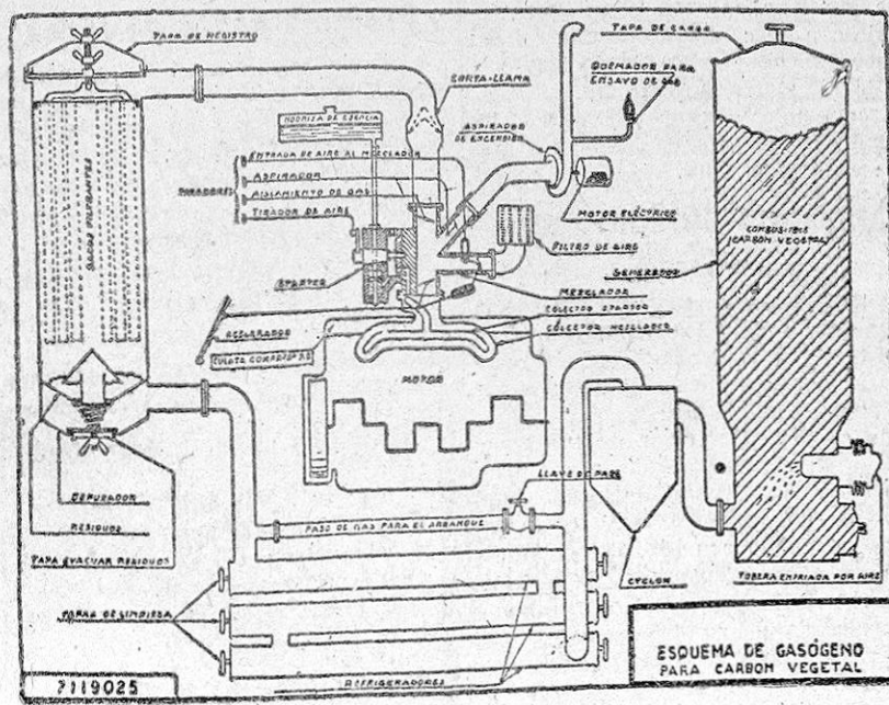
Distribución general del gasógeno
