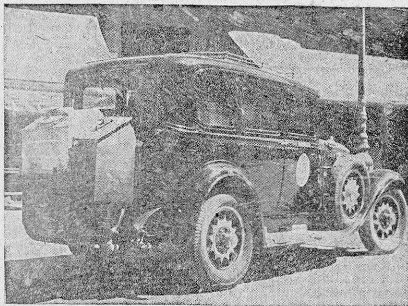
El coche «turismo» con su gasógeno dispuesto a entrar en servicio.
