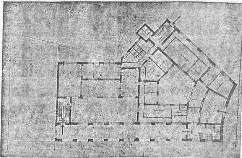
Distribución interior de la planta principal del futuro Palacio de Comunicaciones de Granada.
