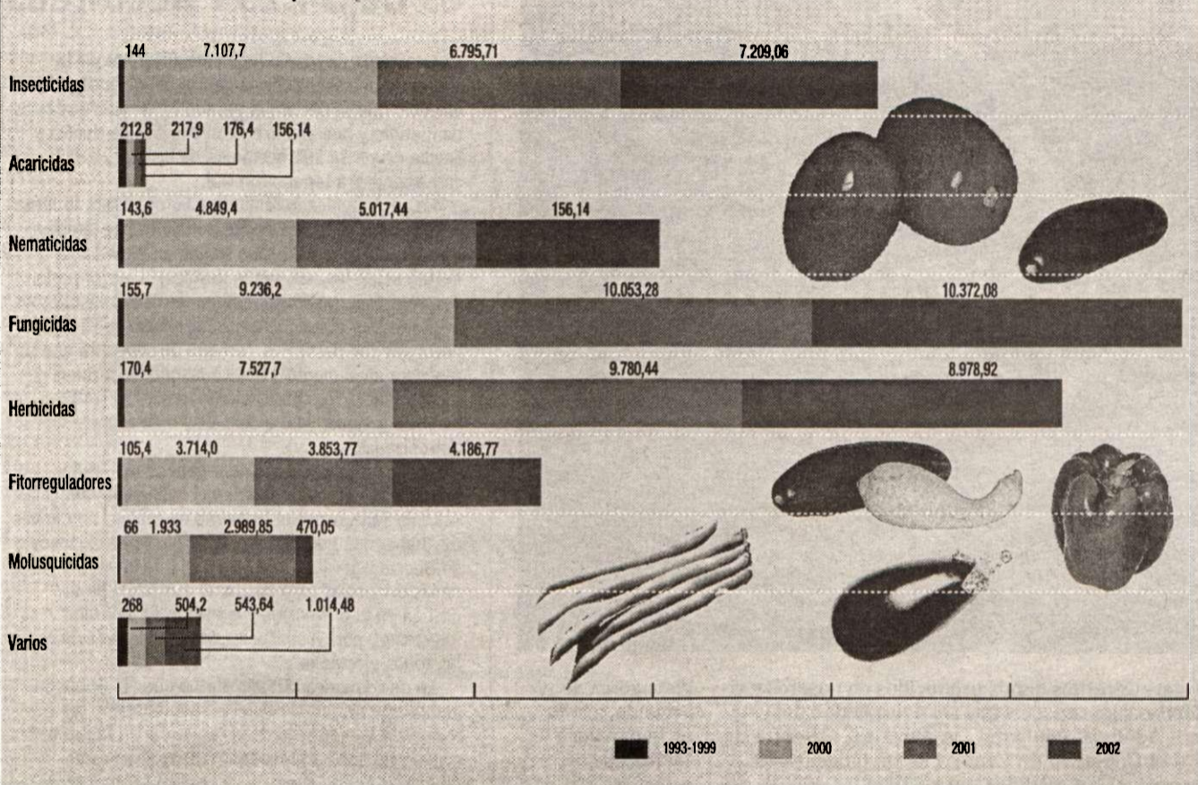
Evolución del consumo de productos fitosanitarios en Andalucía 1993-2002 en toneladas
