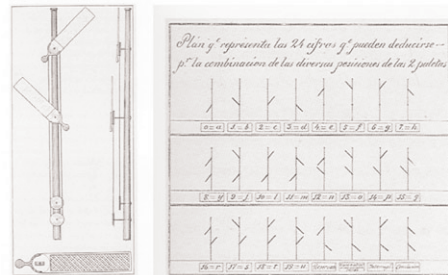
El telégrafo de Hurtado con todas las combinaciones de las paletas
