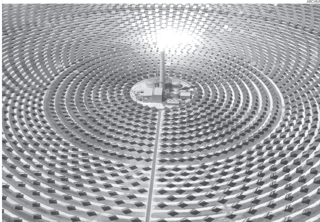
Vista aérea de Gemasolar, que utiliza sales fundidas para mantener el almacenamiento térmico.
