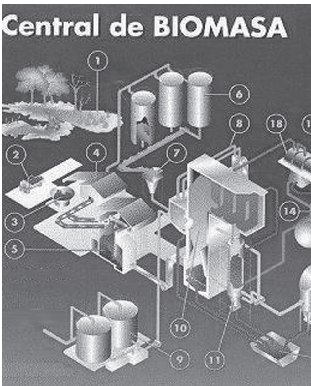
Diseño de una central de biomasa.
