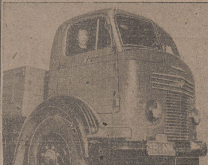
He aquí el nuevo camión inglés "Commer", con una capacidad de carga de cinco a siete toneladas y con motor de 105 caballos. La cabina tiene las mismas comodidades que un coche de turismo, disponiendo incluso de dispositivo para la regulación de la temperatura. (Foto CALPE).
