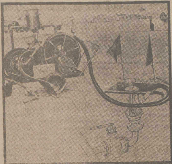
Foto-diagrama de un sistema de boca de riego empleado en los Estados Unidos para reabastecer de combustible a los aviones.
