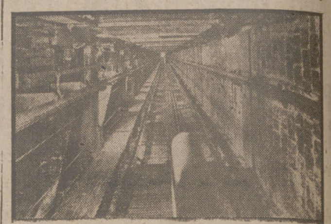
Uno de los dos ejes de ascensores más largos del mundo es este que aquí vemos, el cual mide 245 metros y está instalado en el edificio del Centro Rockefeller, de Nueva York. (Fot. P. A.)
