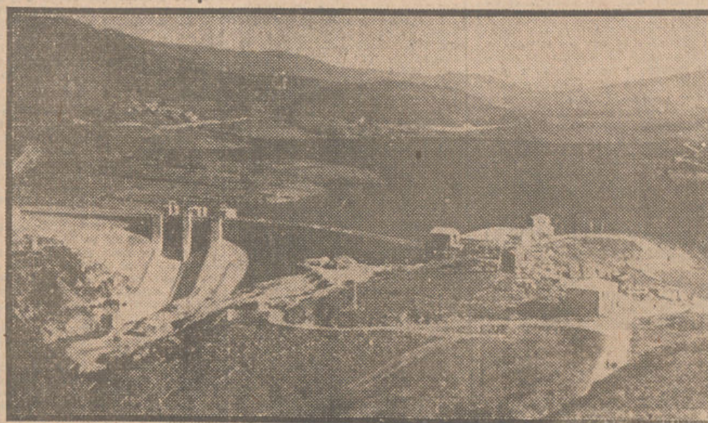
Vista general del nuevo pantano de Las Conchas, en Galicia, recientemente inaugurado por Su Excelencia el Jefe del Estado. (Fot. C-S.)
