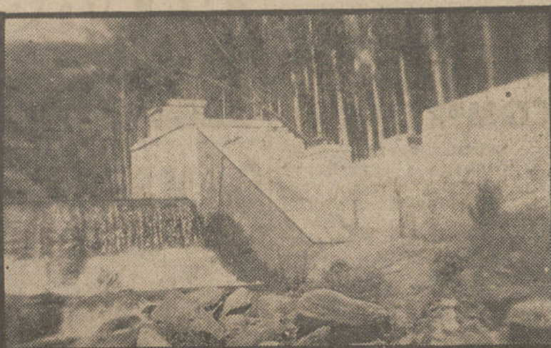
Estación de aforo de la Delegación Hidráulica del Sur de España, en donde está la toma para las aguas potables de Cádiz.
