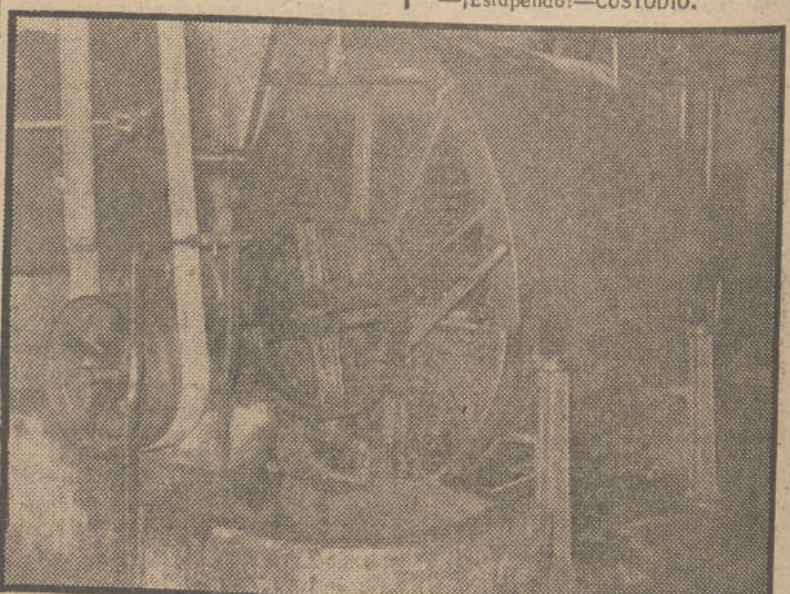
Termo-extractor "Fellú", instalado en la fábrica de aceites "Santa Isabel", de Campotéjar.
