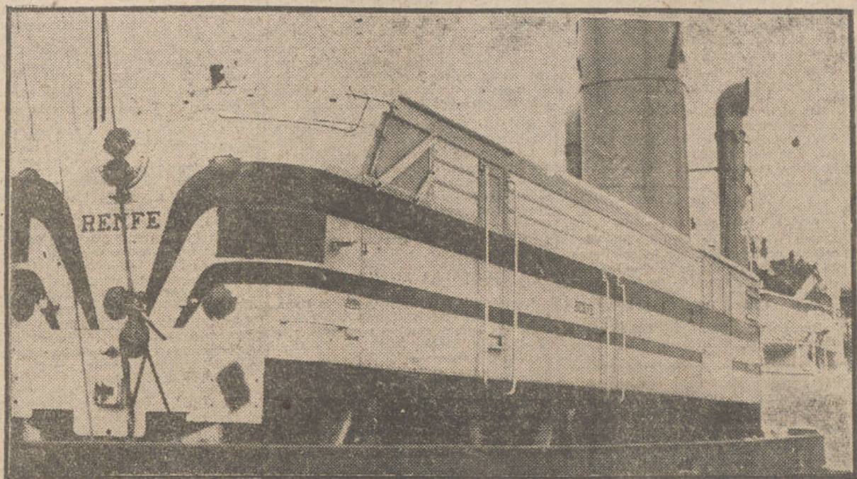
He aquí las dos locomotoras americanas llegadas al puerto de Bilbao, a bordo del vapor "Monte Monjuich", que forman parte del grupo de catorce destinadas a la RENFE. El coste de cada una es de diez millones de pesetas y su peso, de ciento cincuenta toneladas. Poseen producción propia de energía eléctrica por medio de fuel-oil. (Fot. CIFRA GRAFICA.)
