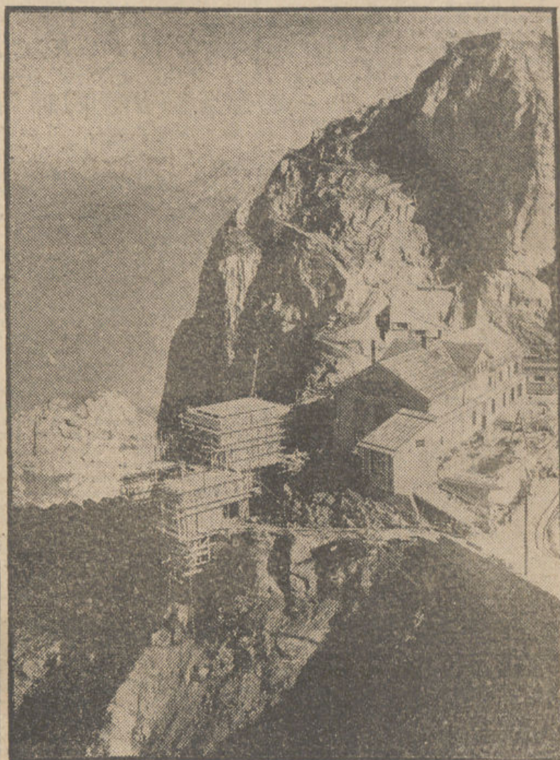
En el monte Piatus, de los Alpes, se construye un funicular de 1410 metros de longitud y con una diferencia de altura de 657 metros, entre Kulm y el Piatus. De este modo, aun en la época invernal cuando esté cortado el ferrocarril y la carretera, se podrá realizar el paso de viajeros. — (Fot. CIFRA GRAFICA).
