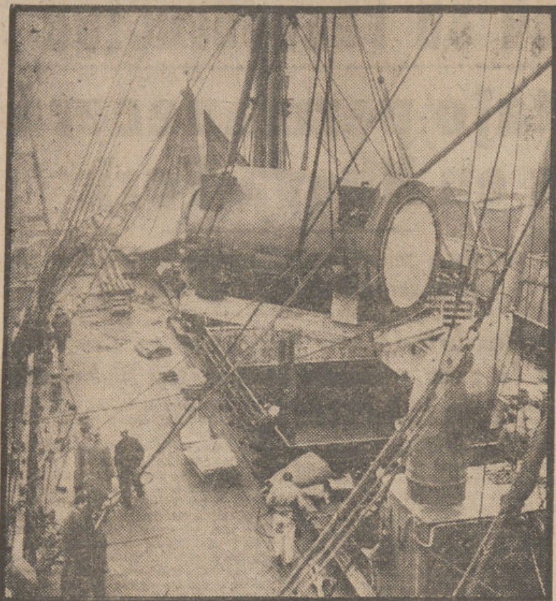
Un momento del embarque en Nueva York, a bordo de buque "Sete", de uno de los elementos de las tres turbinas de vapor con destino a la central eléctrica de Escumbres en Cartagena.—(Fot. A. P.)
