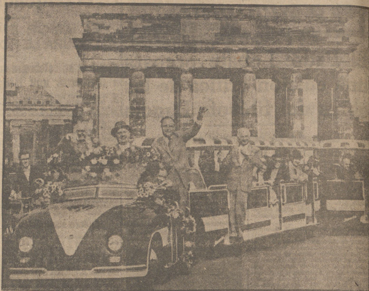
Ingenieros alemanes han diseñado este tren, que no necesita rieles, y que va movido por un motor W.M. Se presentará oficialmente por primera vez en la Exposición alemana que el año próximo será inaugurada en Berlín. En la fotografía vemos la prueba efectuada por el revolucionario tren con asistencia de las autoridades, ante la puerta de Brandeburgo, exactamente al borde del Berlín soviético.
