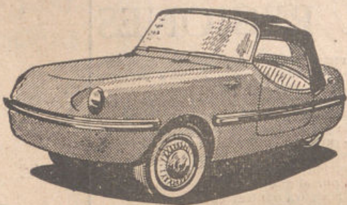
BELCAR (Suiza) Presenta una carrocería en resina sintética y parabrisas muy abombado. Tiene tres ruedas, y tres plazas. Motor monocilíndrico de dos tiempos, 250 cm.3, 11 HP, y 85 Km. h. de velocidad.
