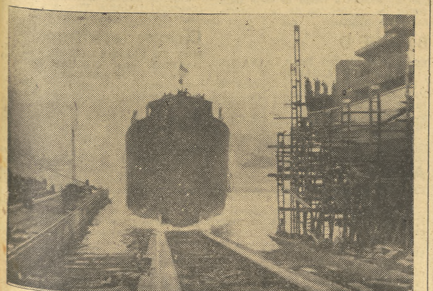
Bilbao.—Botadura del bacaladero «Alicio», cuarto de la serie de seis en cargados por la P. I. S. B. E. a la Constructora Naval.—(Foto Cifra).
