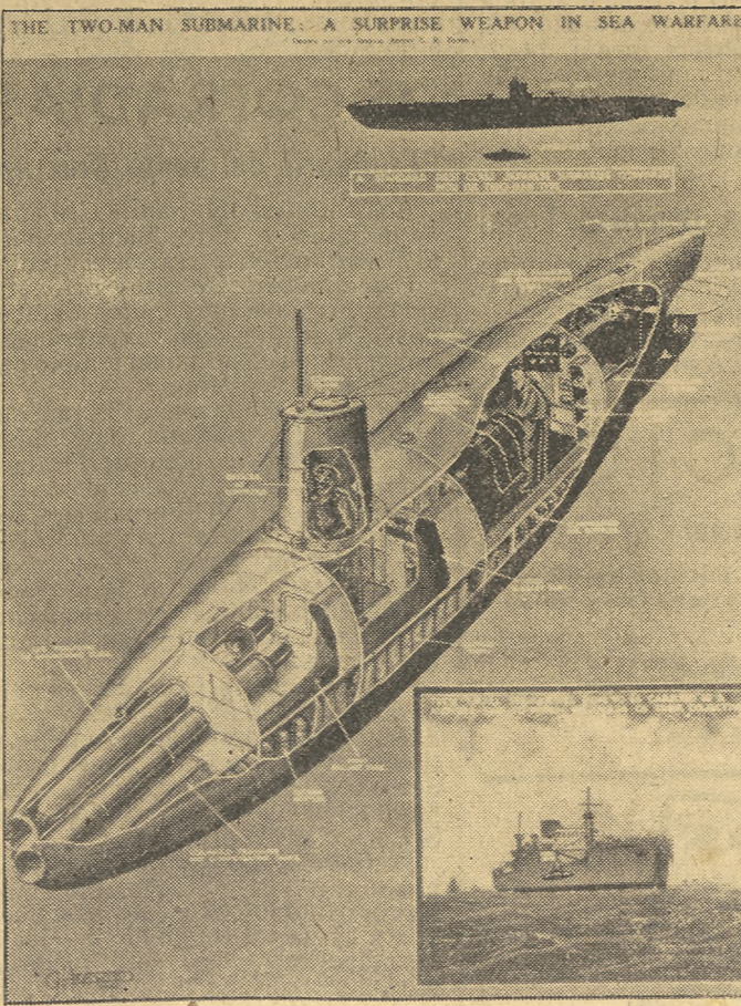
Los éxitos de los submarinos de bolsillo japoneses de una tripulación de dos hombres, han causado gran sensación. He aquí un corte de este buque.—Foto Orbis
