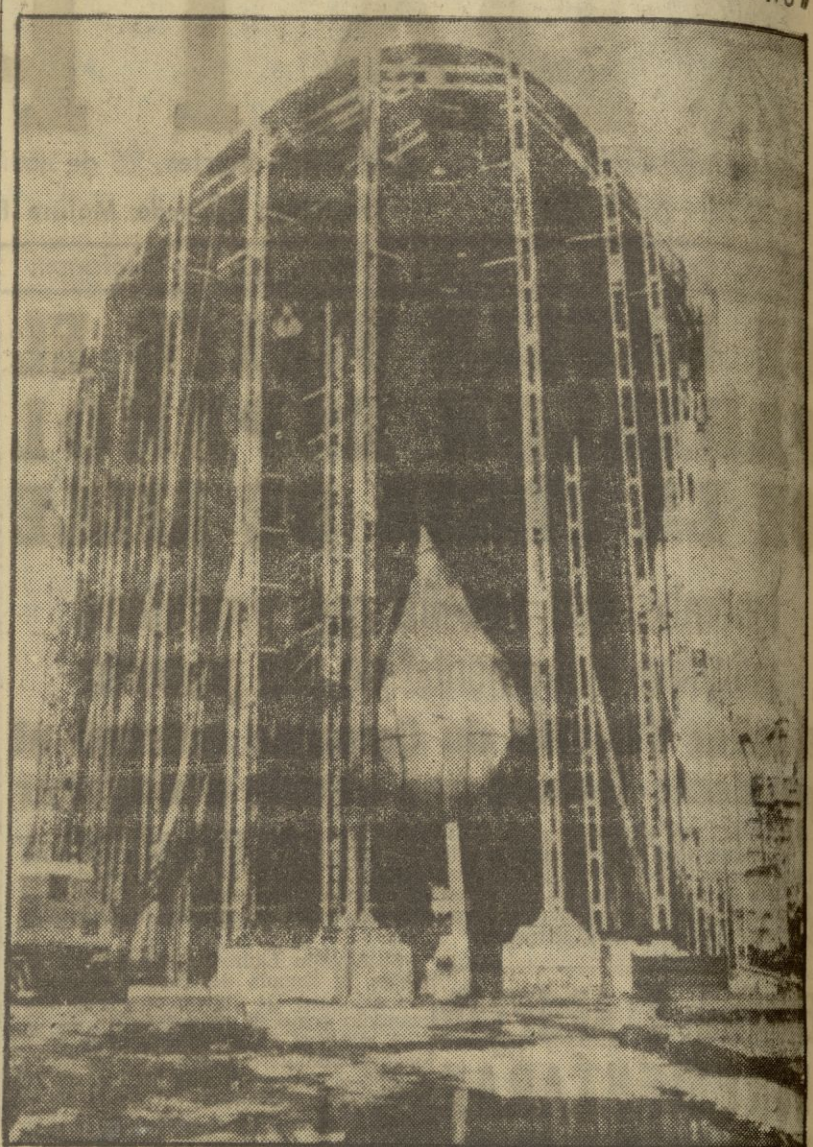
En los astilleros del Noroeste se ultiman los preparativos para la botadura del «Ildefonso Fierro», de 65.000 toneladas de registro bruto, que próximamente será botado en dichos astilleros de la ria ferrolana. Se trata de uno de los barcos de mayor tonelaje construidos hasta ahora en España. En la foto el buque en grada, dispuesto para ser lanzado cuando se retiren los útiles de trabajo que lo rodean. (Foto EUROPA PRESS)
