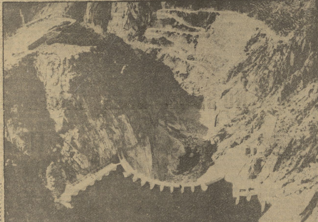
Vista de la grandiosa presa de Aldeavilla. En su interior funciona el ascensor más alto del mundo de un solo recorrido. — (Foto CIFRA)
