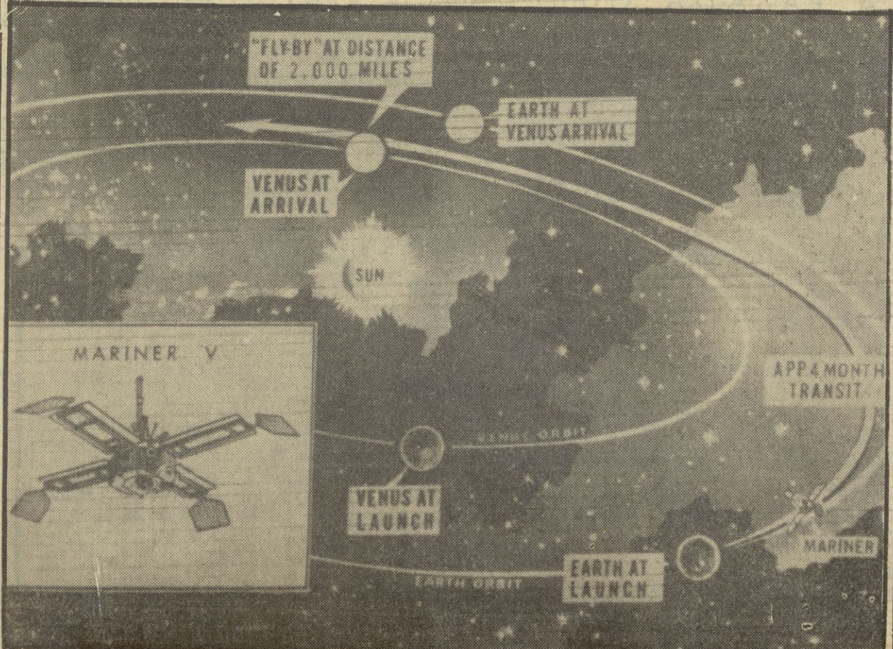
Los Estados Unidos han lanzado un robot espacial «Mariner 5» hacia Venus. El dibujo muestra la trayectoria a seguir hasta alcanzar ese planeta el 19 de octubre y luego regresar a la Tierra. — (Foto UPI-CIFRA)
