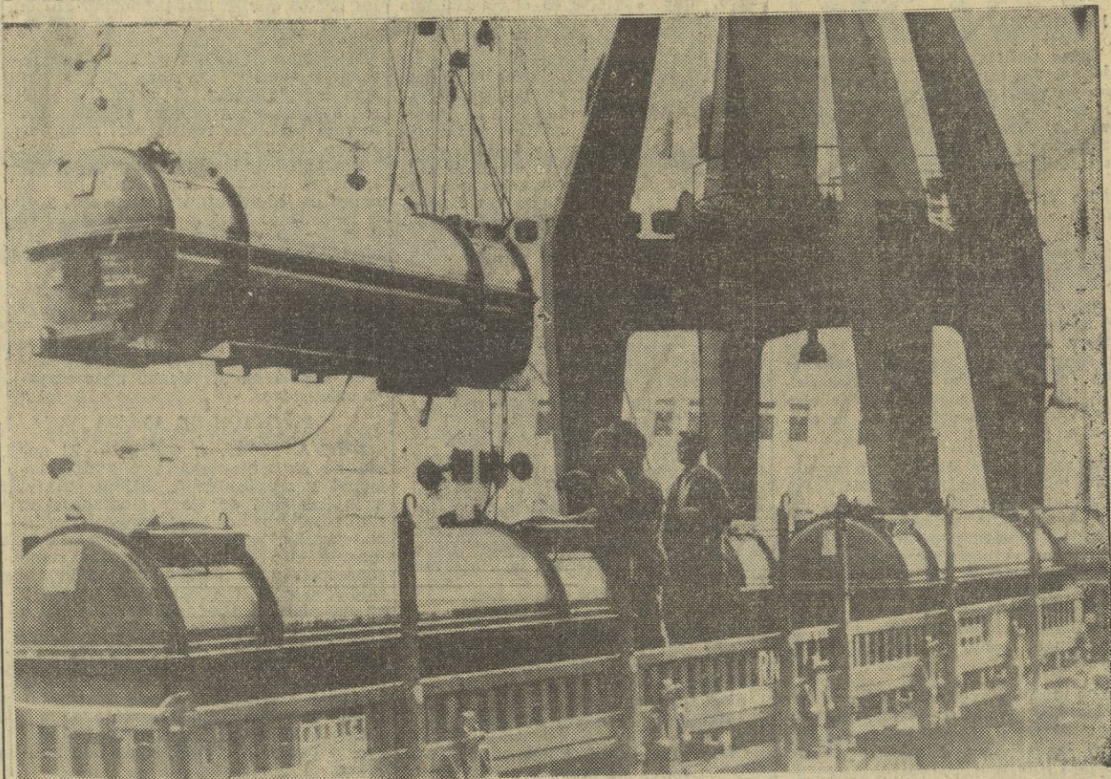
Descarga de la motonave «Covadonga» de las diecisiete toneladas de uranio español enriquecido en los Estados Unidos, valoradas en casi quinientos millones de pesetas y destinadas a la central nuclear de Zorita, en Guadalajara. Estas diecisiete toneladas equivalen a más de un millón y medio de toneladas de carbón. Dicha central estará en funcionamiento comercial el próximo verano.—(Telefoto CIFRA GRAFICA)
