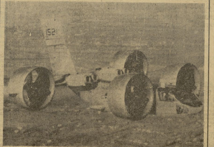
El «X-22A», de aterrizaje y despegue verticales, durante un reciente vuelo de pruebas, en Niagara Falls (Nueva York). El «X-22A» ha completado ya su centésimo vuelo de pruebas con éxito. — (Telefoto UPI-CIFRA)
