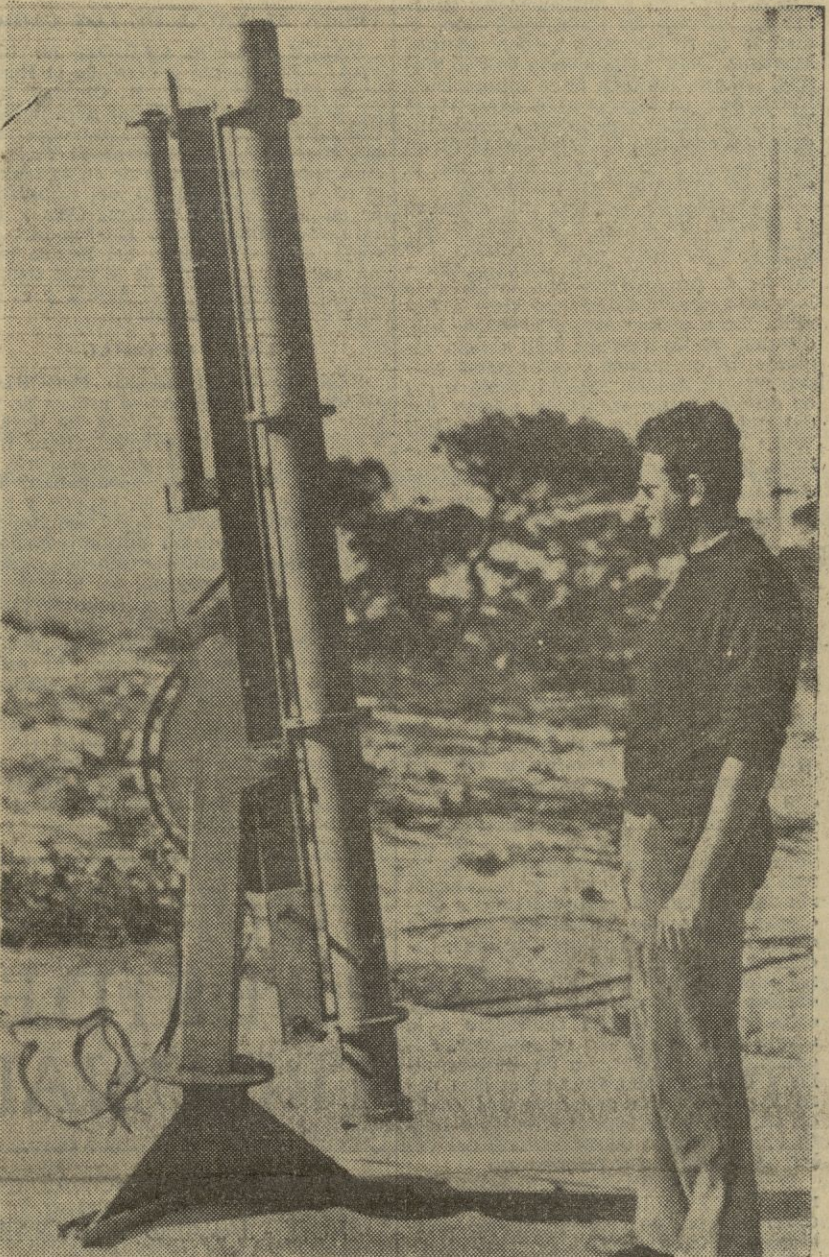
El ingeniero aeronáutico, señor Acárraga, jefe de lanzamiento de la base aeroespacial de Campo Arenosillo (Huelva), ante el cañón de lanzamiento del cohete "Judi Dart", que alcanzó el record de altura de su especialidad, con sesenta y siete kilómetros. (F. EUROPA PRESS)
