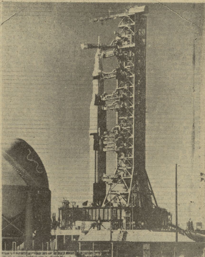
El «Apolo VI», el segundo vehículo espacial sin tripulación del programa Apolo - Saturno, en su plataforma de lanzamiento del complejo 39 de la base de Cabo Kennedy. El vehículo será lanzado para la misión de ejecutar un vuelo de altitud y el reingreso en la atmósfera. (Foto EUROPA PRESS)
