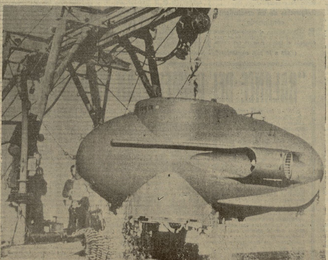
En Santa Bárbara (California), el «Deep Ocean Work Boat» (BOWB), de los Laboratorios de Investigaciones para la Defensa de la General Motors AC Electronics, en el momento de ser izado del agua tras haber contemplado sus pruebas finales con una inmersión de 6.420 pies al fondo marino de la dársena de Santa Bárbara, en el Pacífico. Posee instalaciones ópticas para la visibilidad de los fondos marinos. — (Telefoto UPI-CIFRA)
