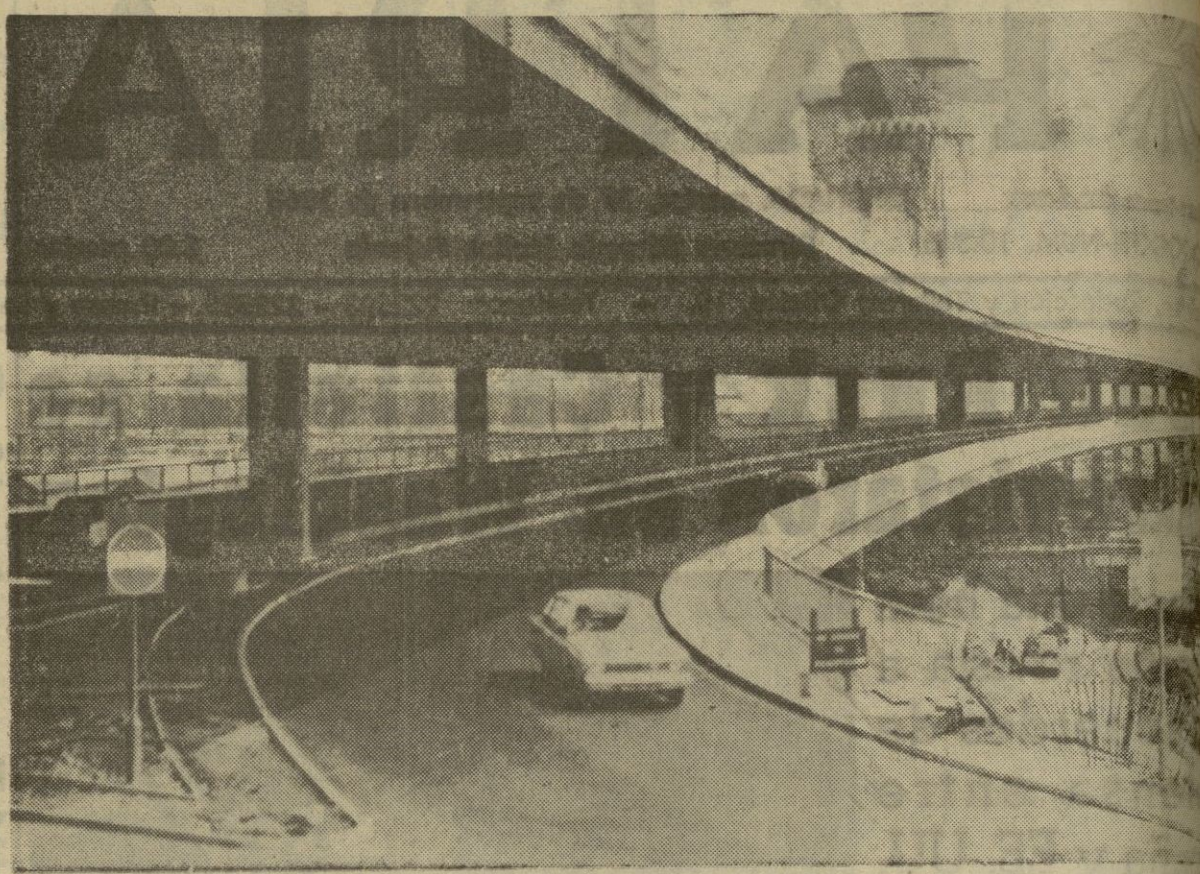
Vista parcial del viaducto de Tinsley, el primero de su clase en el Reino Unido, que cruza el valle del río en Sheffield. El paso superior es de doble calzada, con tres carriles en cada dirección, y el inferior de doble calzada con sólo dos carriles. El viaducto tiene mil doscientos metros de longitud y su importe ha sido de cuatro millones y medio de libras.—(Foto EUROPA PRESS)
