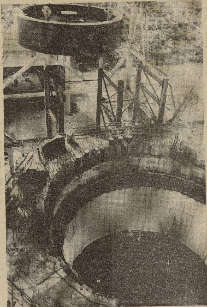
Colocación de la "tapadera" del reactor de la central eléctrica de energía nuclear de Vandellós (Tarragona). En 1972 se espera que entre en servicio esta central, la tercera española de su género.
