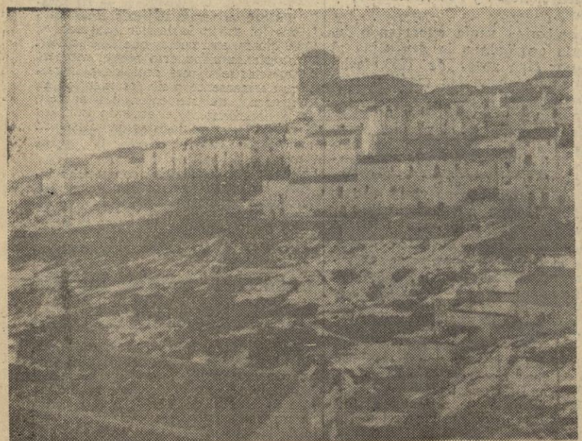
Vista parcial de Alhama, en la que puede apreciarse aún restos de la nieve caída hace unos días.
