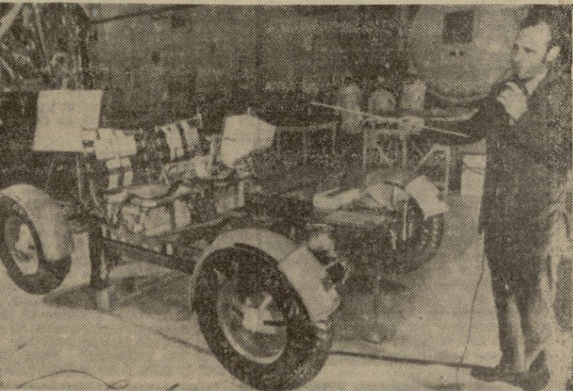
Lindsey Bolton, ingeniero proyectista del vehículo lunar, explica el diseño junto a un modelo del mismo. El vehículo será usado para transportar a los cosmonautas del "Apolo XV" por la Luna, durante su misión, prevista para el 26 de julio. — (Telefoto CIFRA)
