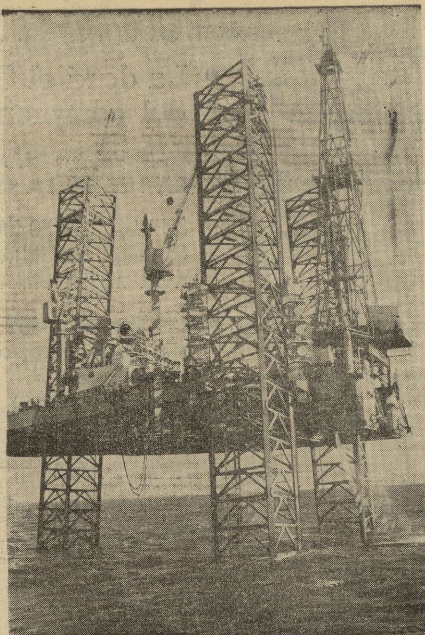
Esta es la plataforma «Chaparral», con la que se realizan prospecciones petrolíferas en la costa mediterránea española, y que ha permitido un importante hallazgo. — (Foto EUROPA PRESS)
