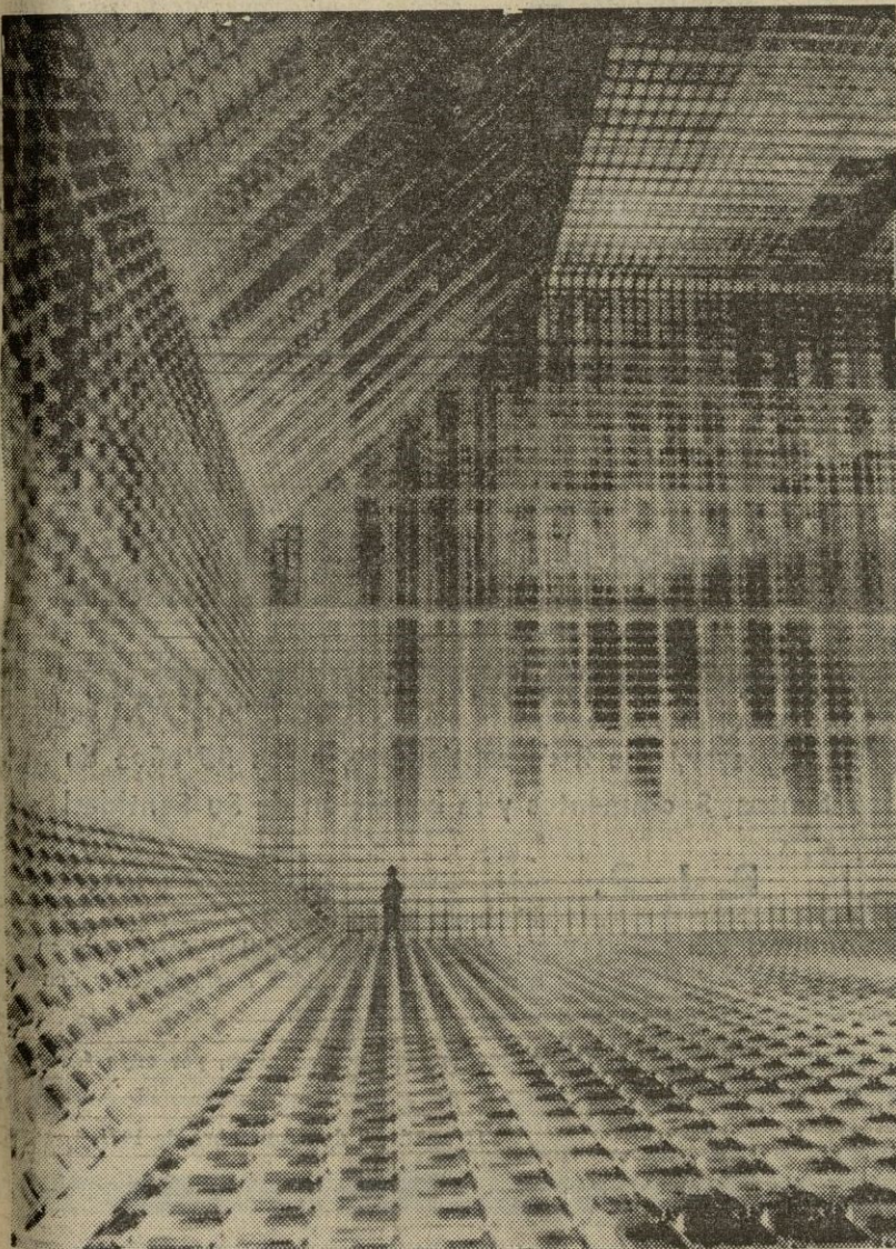
Esta es la impresión que ofrece este trabajador en uno de los tanques de almacenamiento de metano del buque francés «Descartes», que va a ser puesto en servicio. El buque cargará 50.000 metros cúbicos de gas líquido. — (Telefoto A P-EUROPA PRESS)
