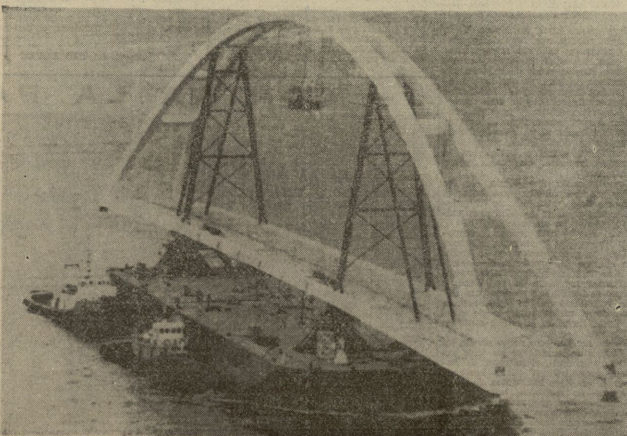
En la foto, un remolcador arrastra una gran plataforma con un puente de 850 toneladas, desde el puerto de Ichihawa al puerto de Toba, doscientas millas al Suroeste de Tokio. El puente tiene 195 metros de largo y 8,25 de ancho y será instalado en una autopista cerca de Toba. — (Telefoto CIFRA GRAFICA-UPI)
