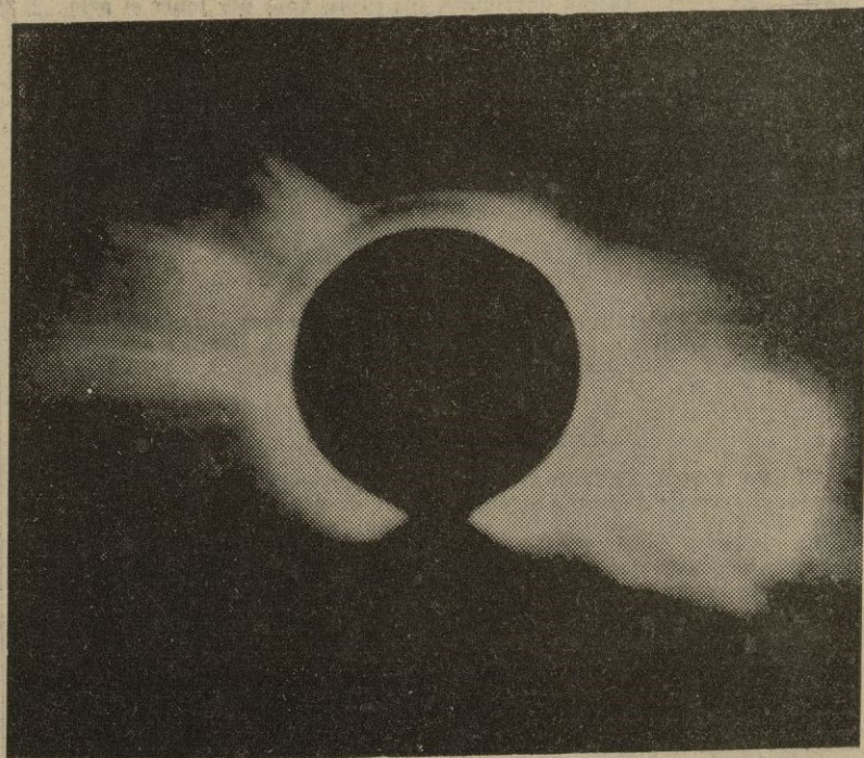
Esta foto, captada por el «White Light Coronagraph» a bordo del «Skylab» el pasado día 10 de junio, muestra una erupción solar que abarca 220 veces el diámetro de la Tierra, expandiéndose hacia el espacio a una velocidad de 1.600.000 kilómetros por hora. Este tipo de erupciones son resultado de la intersección entre materia solar y campos magnéticos en torno al Sol. — (Telefoto CIFRA GRAFICA-UPI)
