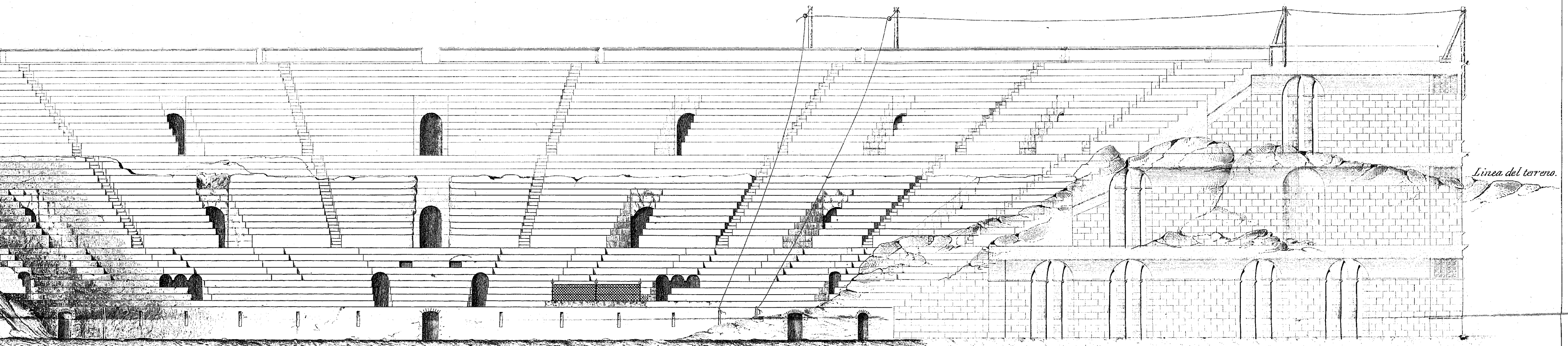
CORTE LONGITUDINAL POR E.O. PARTE SUR
