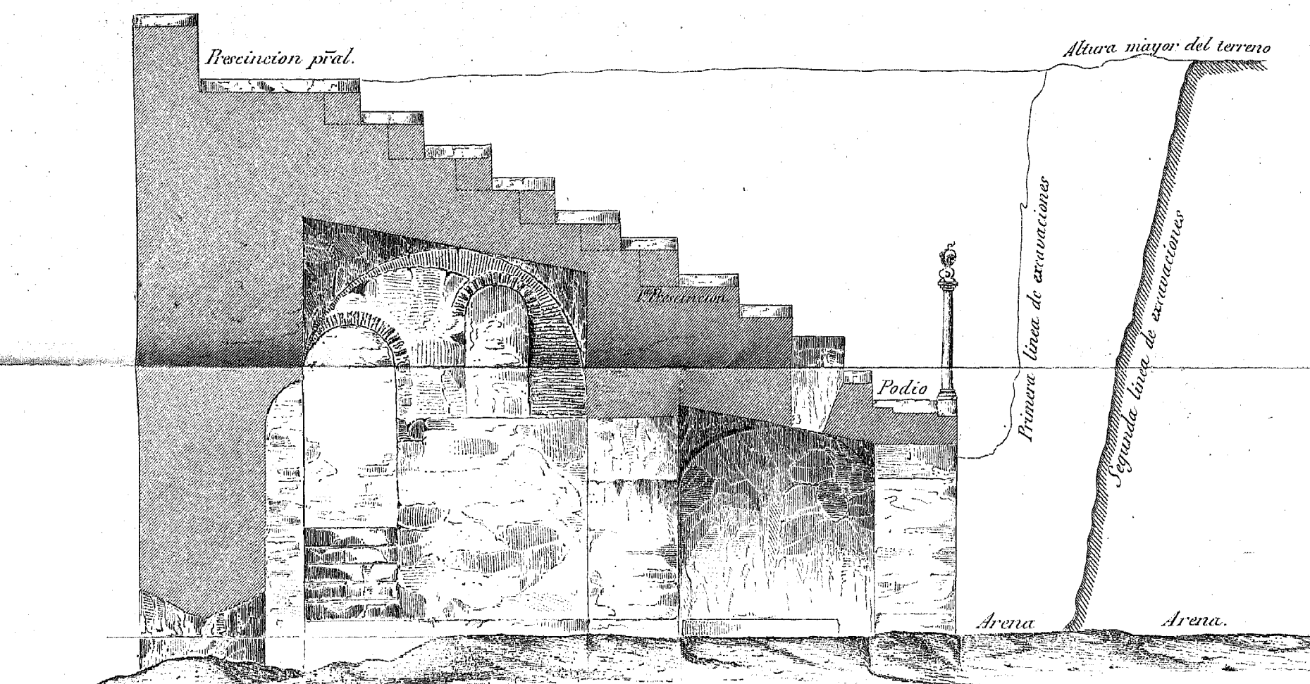
DETALLE T DEL PERFIL N. S. (Vase su parte correspondiente)
