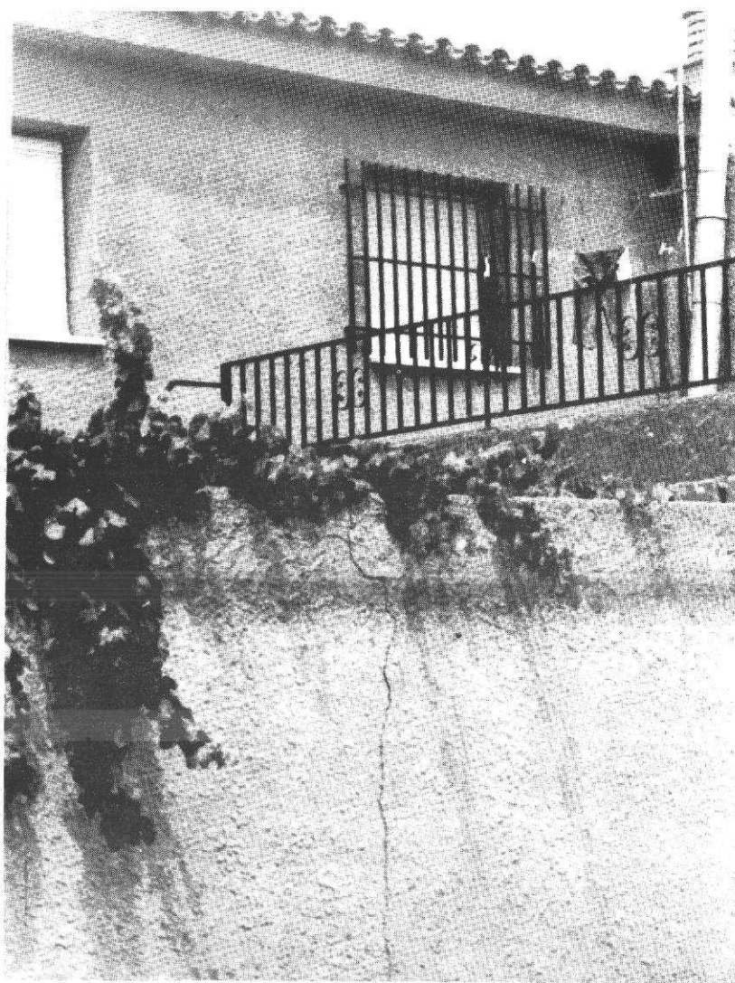
Fachada posterior de una vivienda donde se aprecia una fisura.
