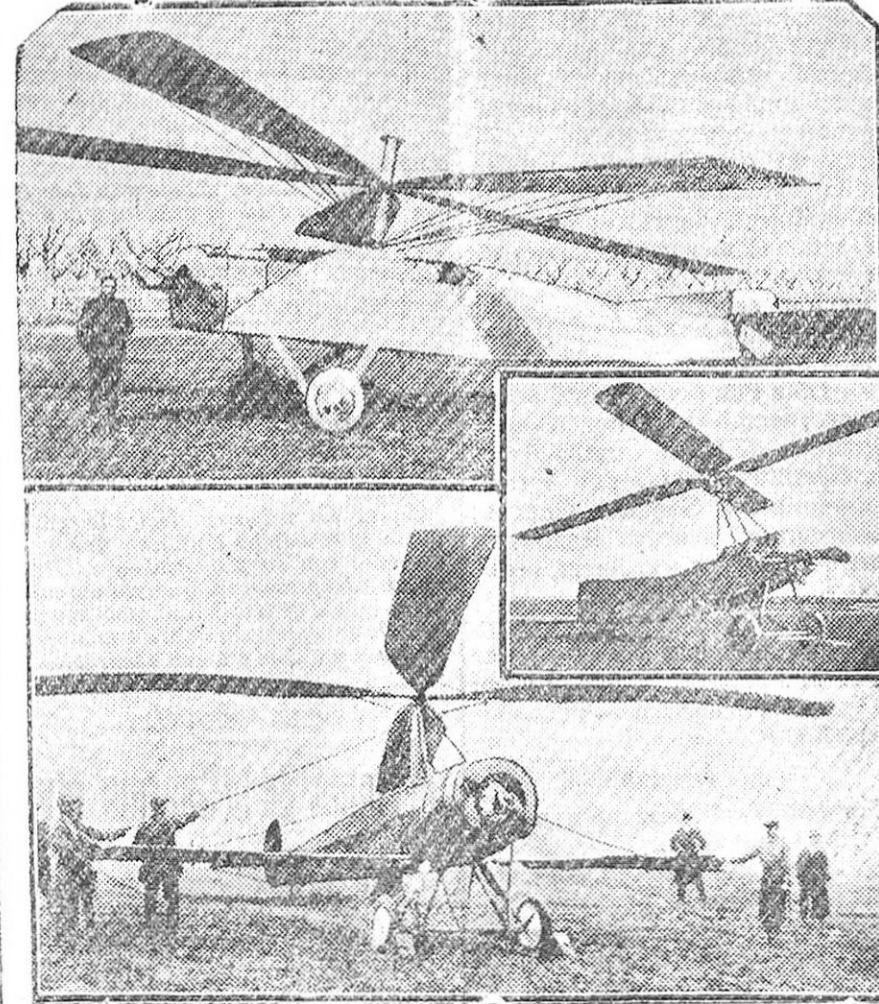
Los tres principales modelos de autogiros construidos por el señor La Cierva. 1.º aparato que señaló al inventor modificaciones necesarias importantes; 2.º primer autogiro en que se logró de pagar de tierra y realizar vuelos en línea recta a medio metro de altura; 3.º estado actual del invento, modelo con el que se realizaron las definitivas pruebas en España e Inglaterra.
