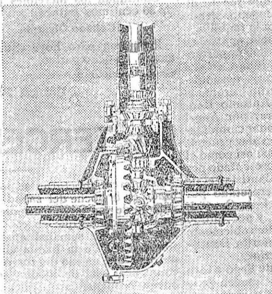
Nuevo puente trasero con piñón de ataque
