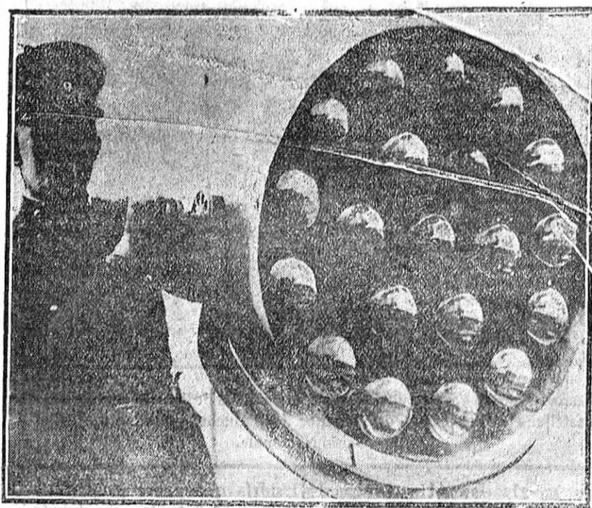
Nuevo proyector para la aviación, que ha empezado a funcionar en el aeródromo de Berlín. Está compuesto por veinte pequeños proyectores muy potentes, y no sólo indica a gran distancia el campo de aterrizaje a los aviones que vuelan de noche, sino que al propio tiempo iluminan también el mismo terreno de aterrizaje.
