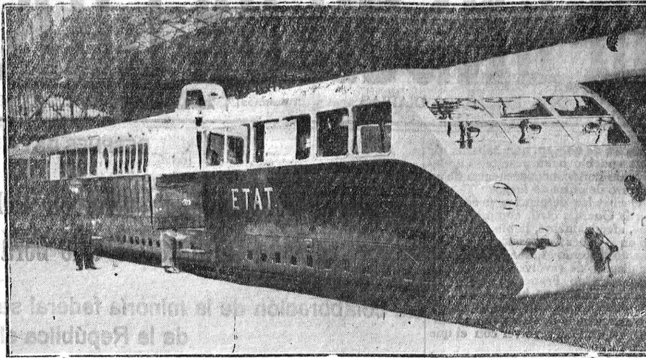
El automóvil sobre rieles, movido por cuatro motores de 220 caballos, que ha realizado durante sus ensayos una velocidad de 275 kilómetros por hora y que puede transportar cincuenta viajeros. Este verano circularán coches de este tipo entre París y Deauville, cubriendo la distancia en dos horas.
