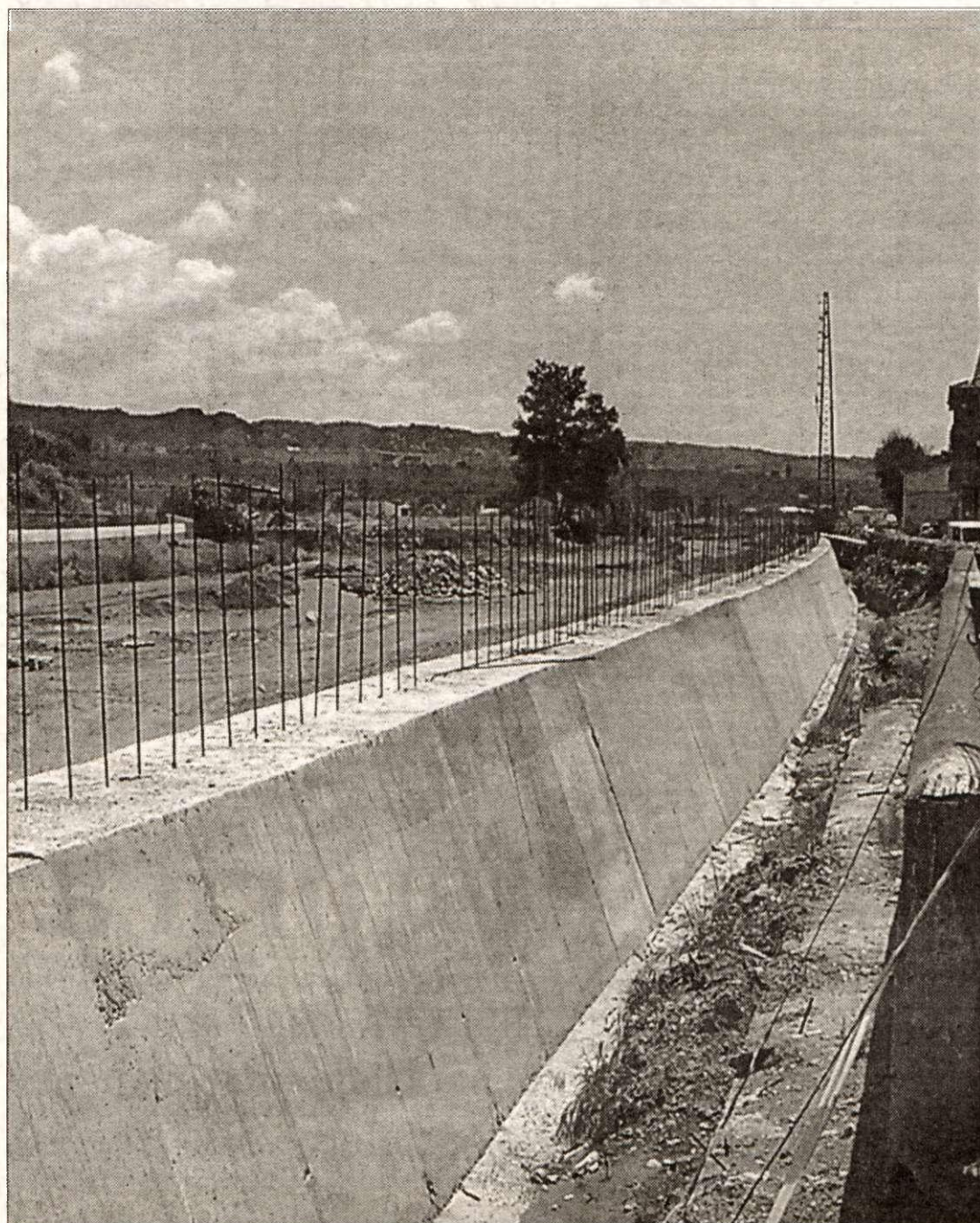
Nuevo muro de contención del río Guadix.
