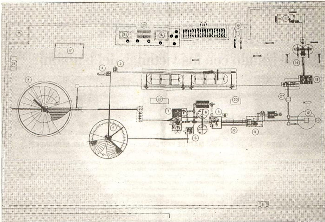
Plano del circuito interno del proyecto de la fábrica de cemento.
