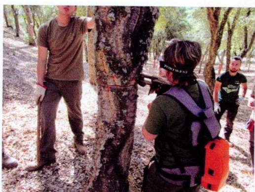
Desbornizando con máquina descorchadora Coveless 3C18
