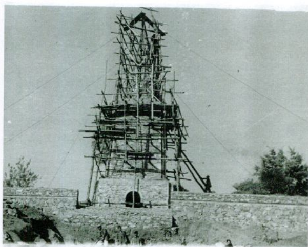
Plano general de la obra. Se observa el sistema de apuntalado y atirantado del sistema de andamiaje de madera, anclados al suelo. (Fotografía cedida por la familia Pinedo Caballero)
