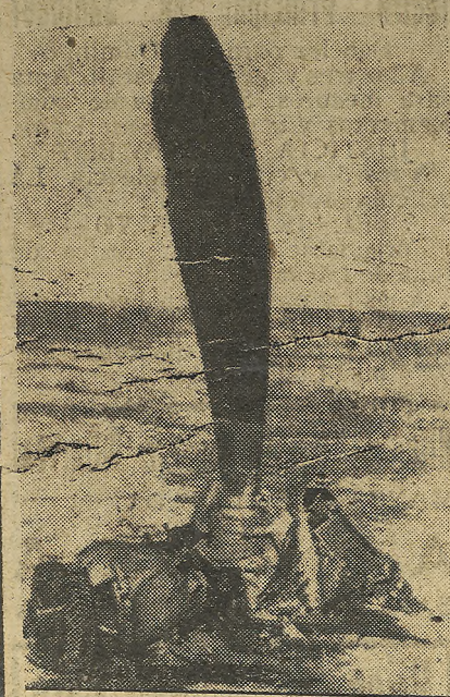
La fotografía muestra una hélice y parte del motor; la otra parte fué a parar a unos doscientos cincuenta metros de distancia. (Foto Trasocéano).
