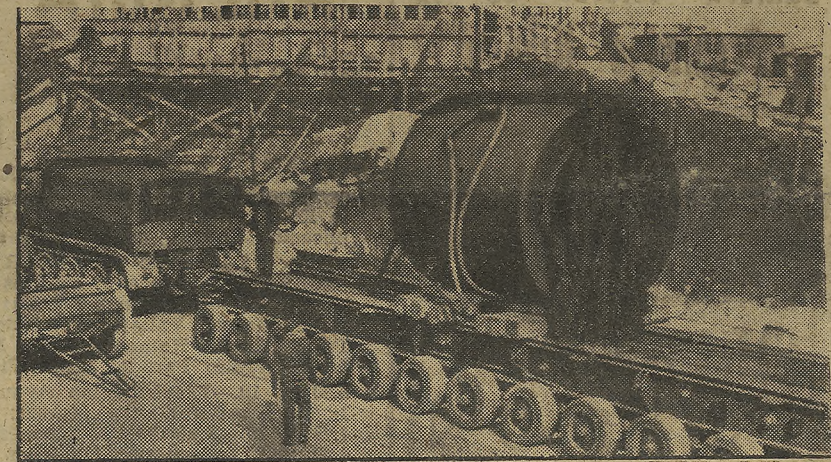
Pieza de una batería pesada la cual es transportada por medio de un potente vehículo, para proceder al inmediato montaje de uno de estos cañones en la costa del Canal. (Foto Trasocéano)
