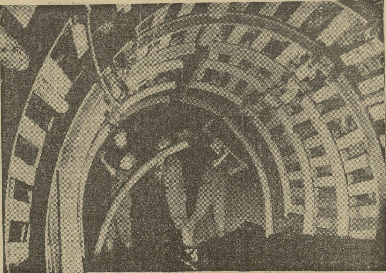
PREPARANDO ENTIBADO METALICO
