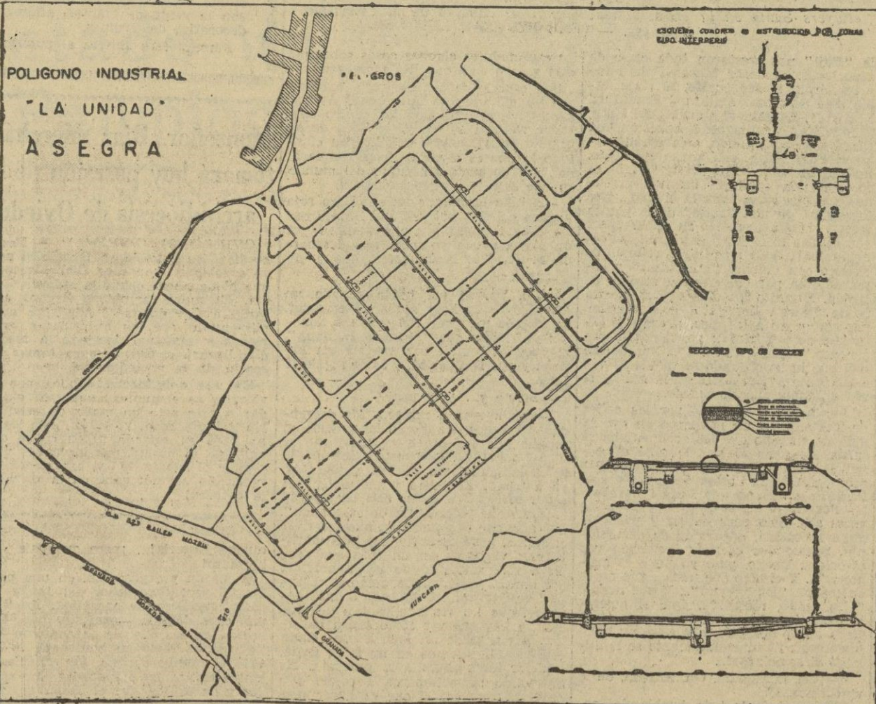
En este plano se recoge el trazado de la urbanización del polígono industrial de la Asociación Sindical de Empresarios de Granada, cuyas obras dieron comienzo ayer, en presencia de las autoridades. En la parcelación efectuada se han dispuesto calles de acceso al conjunto desde la carretera de Madrid, con la que limita. La urbanización comprende pavimento, redes de aguas y servicios comunes.
