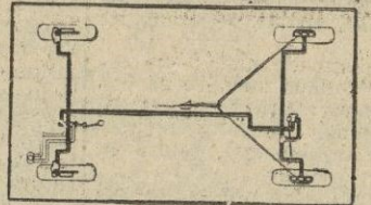
Circuito de frenos dobles e independientes. Corrector de frenada sobre las ruedas posteriores.
