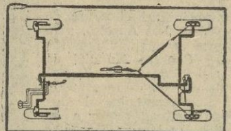
Circuito de frenos dobles e independientes. Corrector de frenada sobre las ruedas posteriores.
